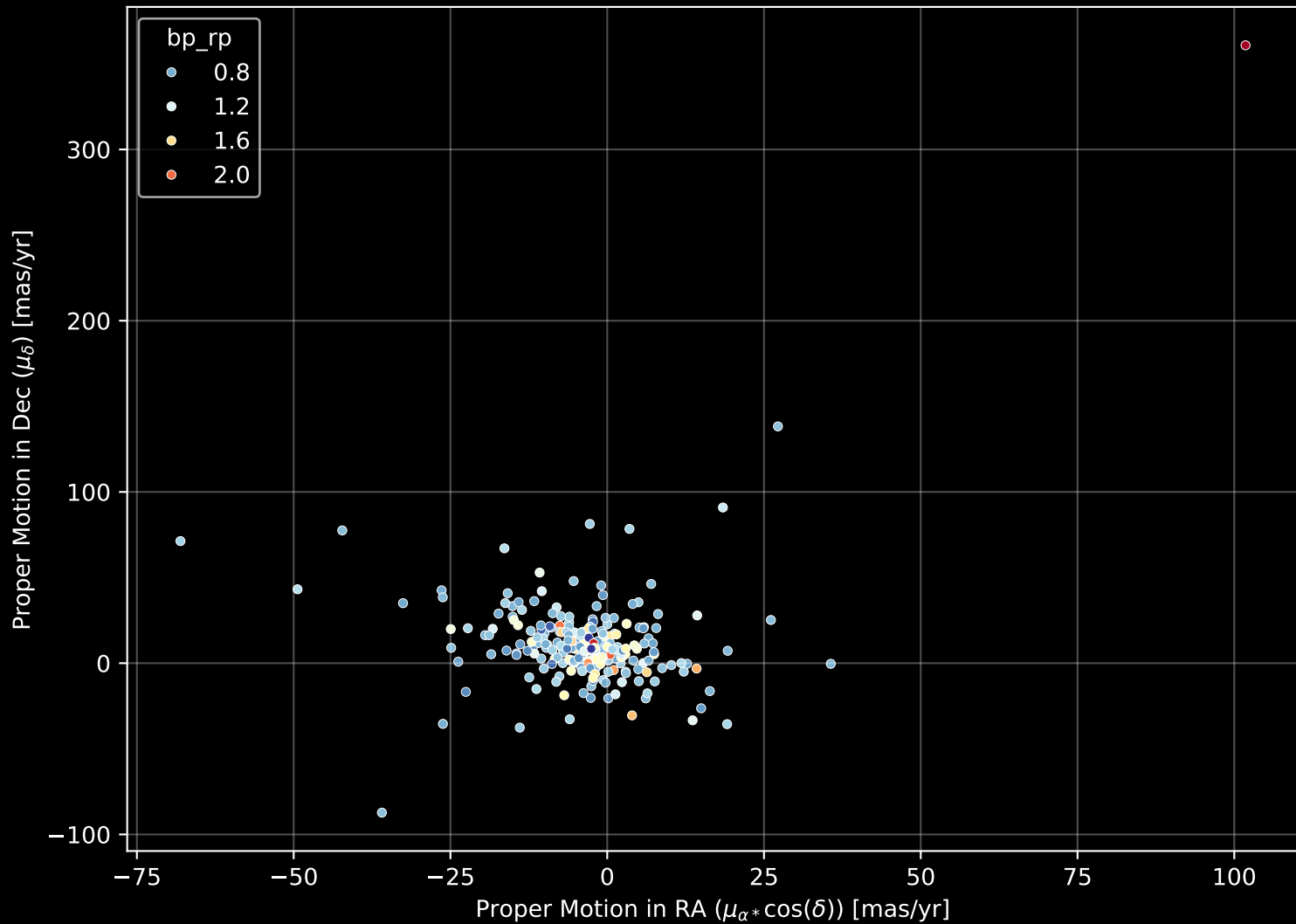
GALAH DR4 Field: [7199] Proper Motion Diagram (n= 254)
