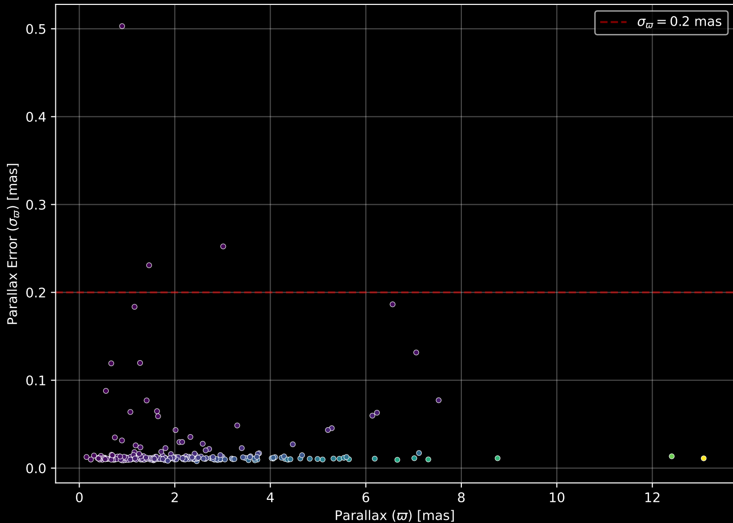
GALAH DR4 Field: [7199] Parallax Quality (n= 254)
