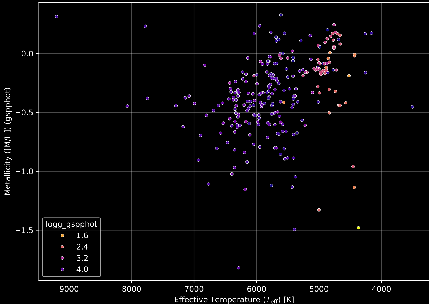
GALAH DR4 Field: [7199] Stellar Population Parameters (n= 254)
