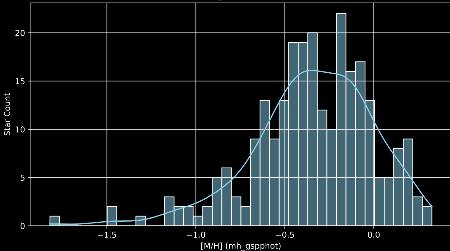
GALAH DR4 Field: [7199] [M/H] (mh_gspphot) (n= 254)
